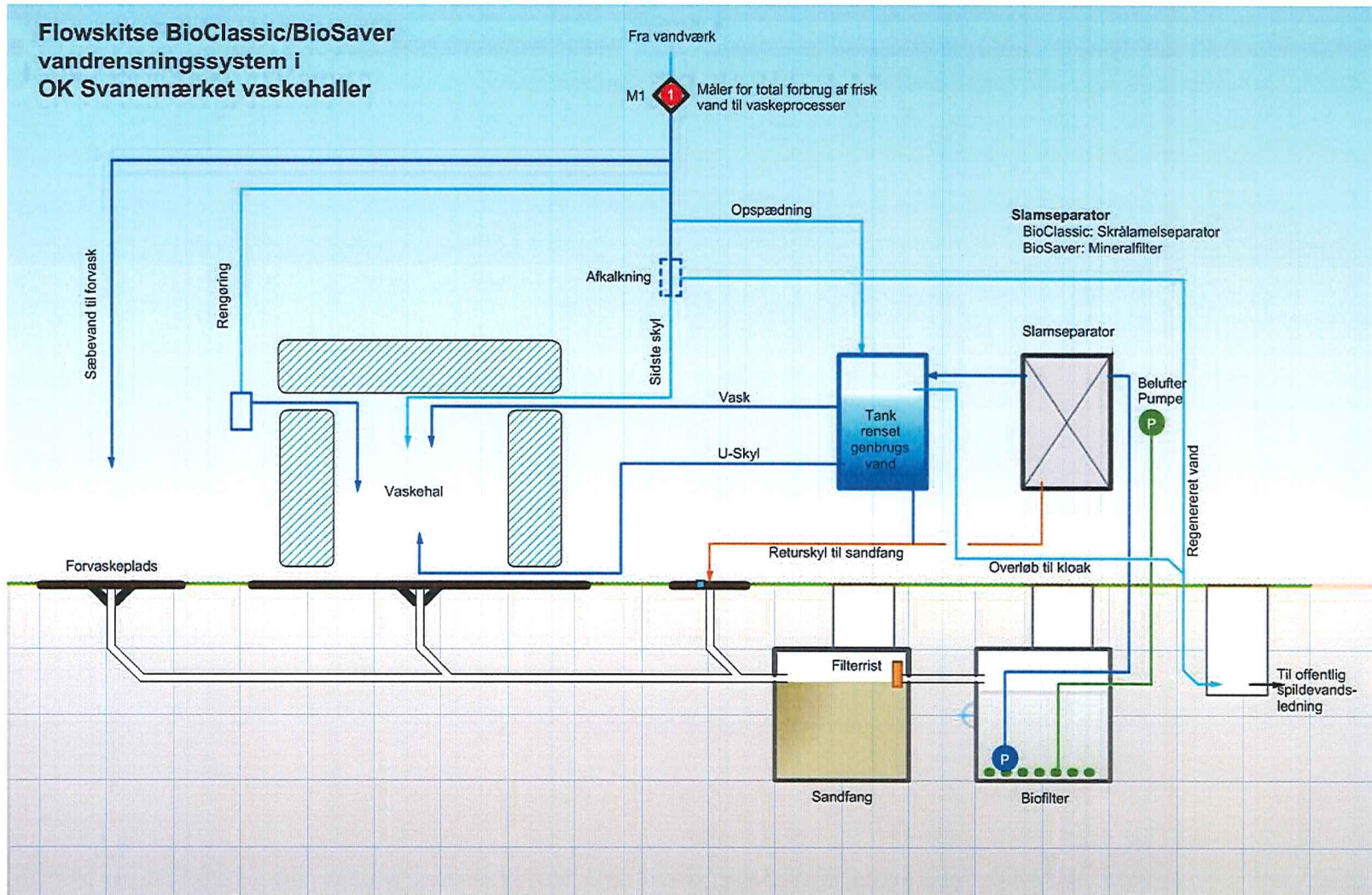
Fig. 2.1 Principskitse
