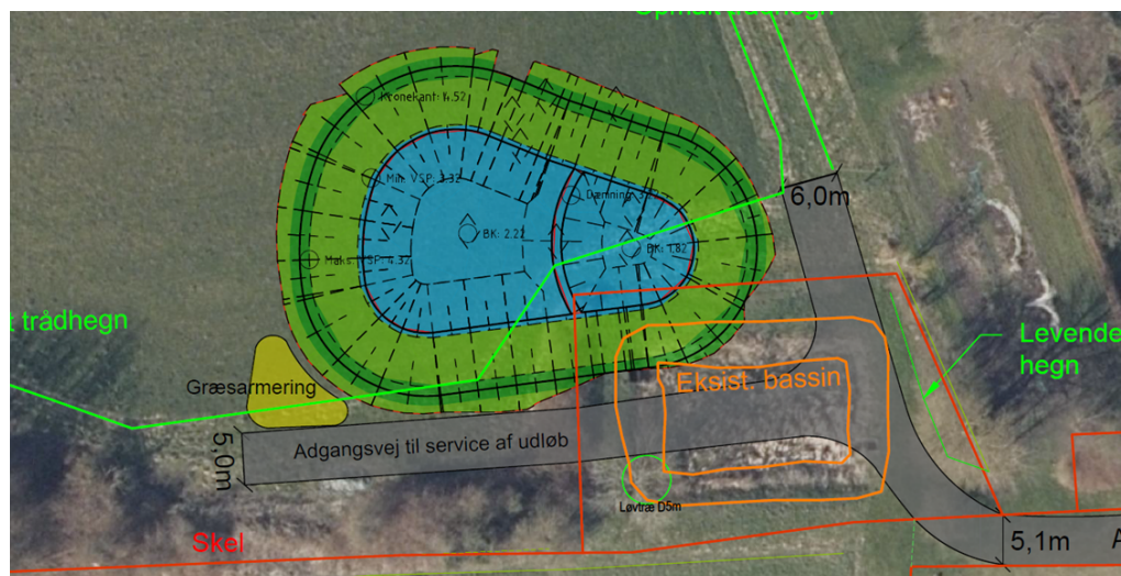
Figur 2: Udformning og placering af regnvandsbassinet.
