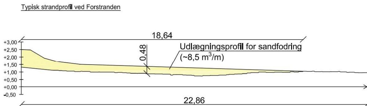
Figur 4-7 Typisk strandprofil ved Strandbyvej, baseret på topografisk data fra SCALGO ( www.scalgo.com ).
