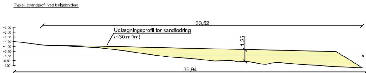
Figur 4-5 Typisk strandprofil ved bølgebrydere. Baseret på opmåling, se underfigur c i Figur 3-7.
