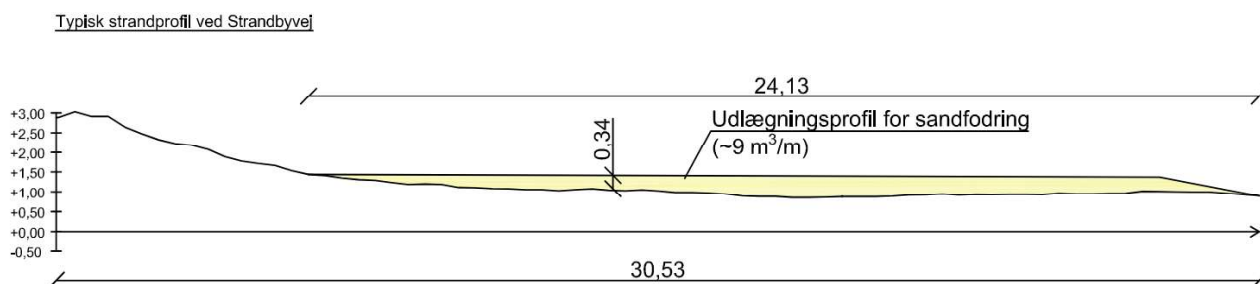
Figur 4-6 Typisk strandprofil ved sydlige bølgebrydere. Baseret på opmåling, se underfigur f i Figur 3-7.
