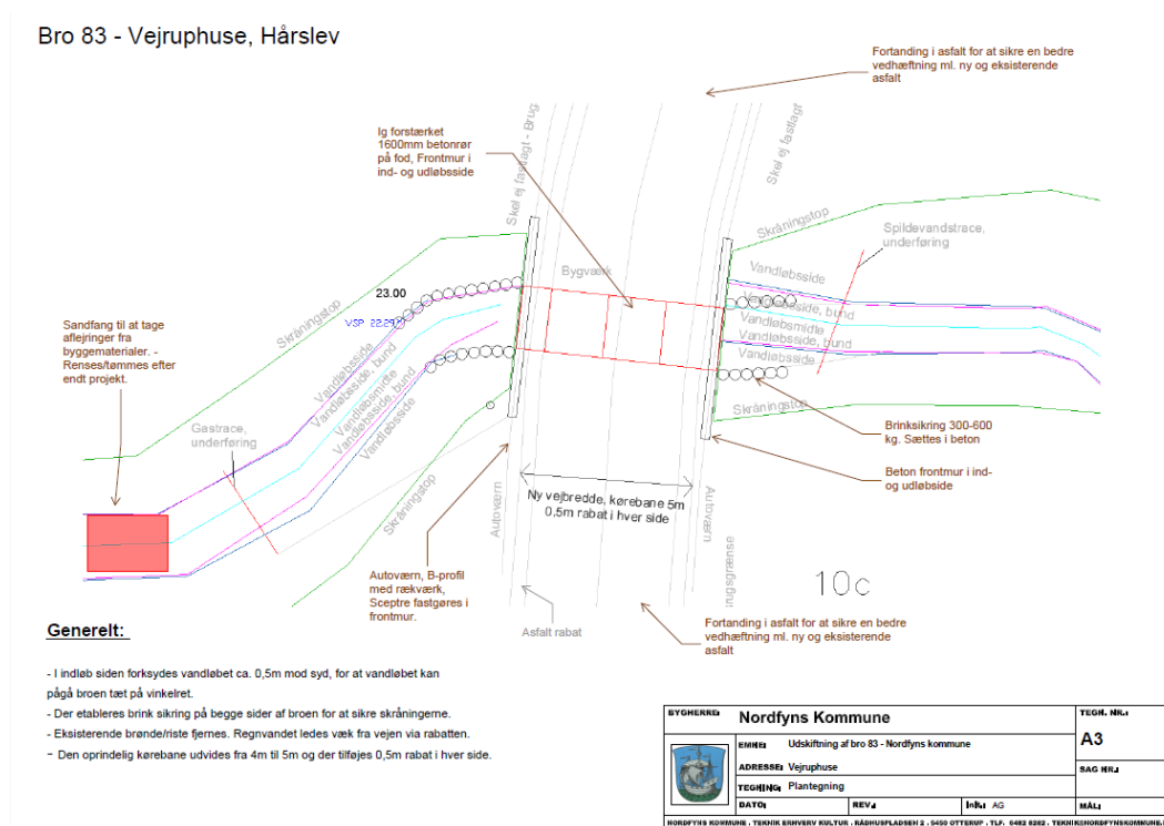
Figur 1: Ny vejbro
