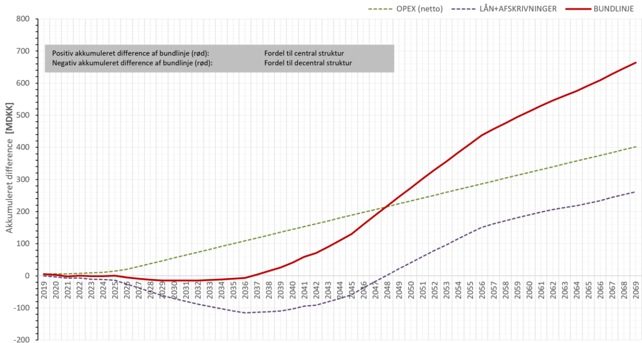
Figur 30 Akkumuleret TOTEX kurve for differencen mellem den decentrale struktur og en centraliseringsstruktur, 40 årig periode
