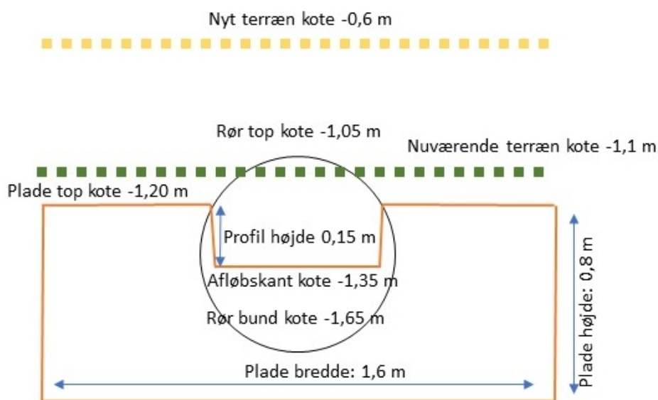
Figur 4: Principskitse for afløbskanten
