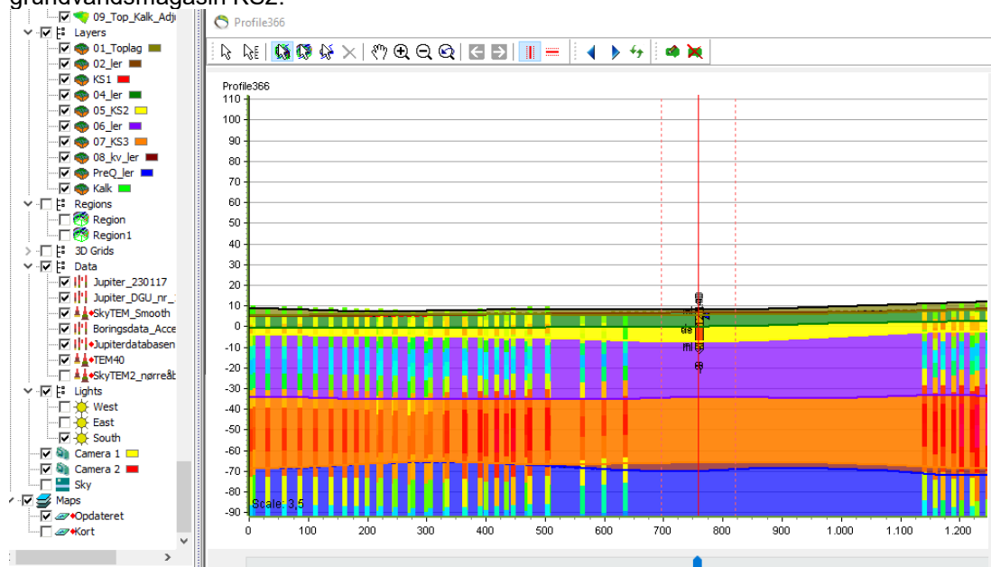
Figur 1: Kort over jordlag ved transformerstation. Transformerstationen er markeret med en rød søjle. Der har tidligere været en boring på ejendommen den er nu sløjfet. Der ses et ca. 10 meter tykt morænelag inden det regionale grundvandsmagasin KS2 mødes.
