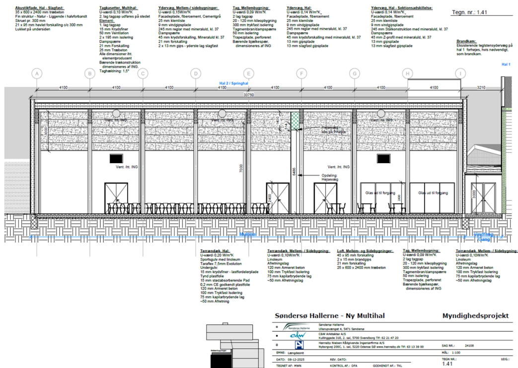
Figur 4. Længdesnit af multihal
