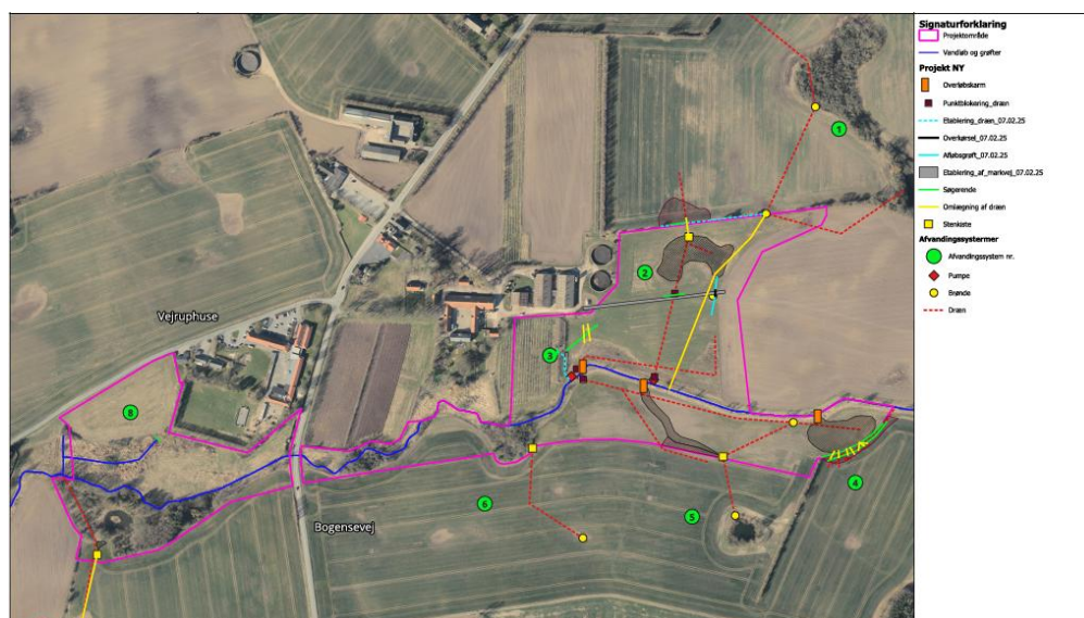
Figur 1 Anlægsteknisk oversigt.
