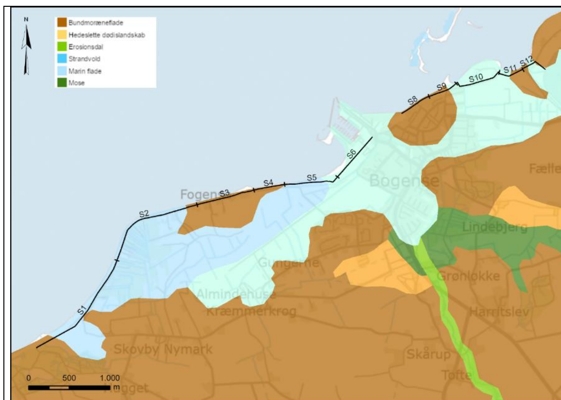
Figur 14-2: Geomorfologien i og omkring projektområdet (GEUS, 2023).
