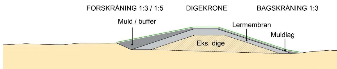
Figur 3 Principskitse for løsning med jorddige
