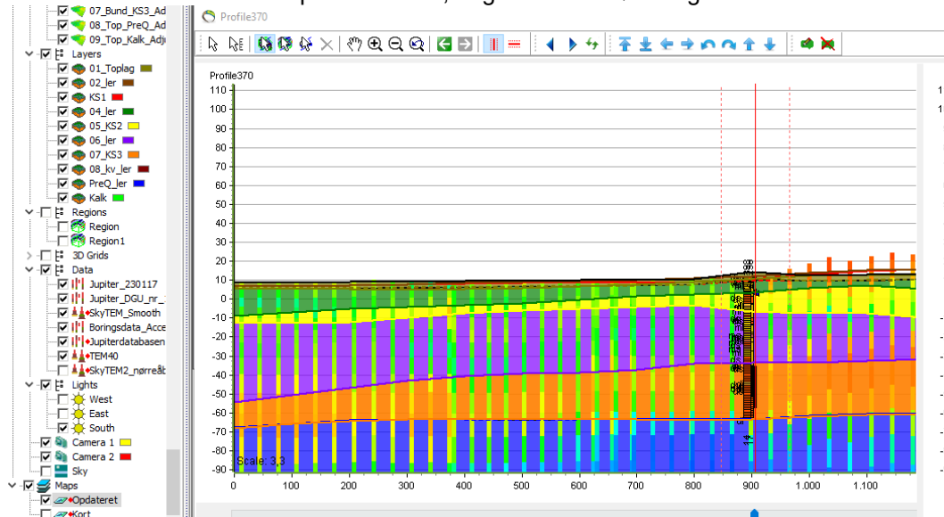
Figur 2: Geologisk profil af boring DGU nr. 127.398. Vest til venstre og øst til højre
